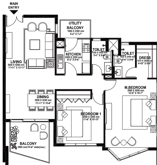
TYPE MR1A (2BR)
